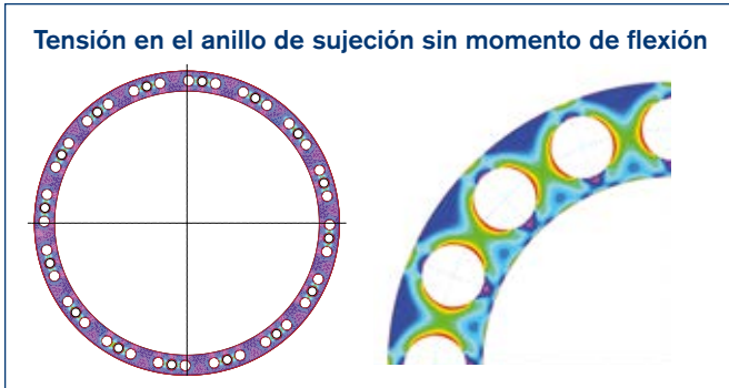
Tensión en el anillo de sujeción con momento de flexión
