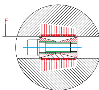
Presiones de superficie con momento de flexión
