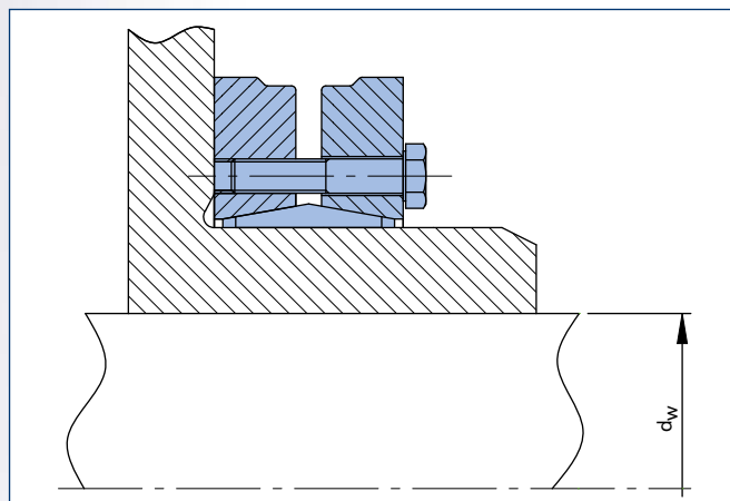
RINGFEDER® Anillos de contracción RfN 4061 • Esquema de montaje
