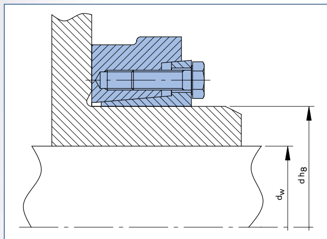
RINGFEDER® Anillos de contracción RfN 4161 • Esquema de montaje
