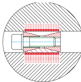
Presiones de superficie sin momento de flexión
