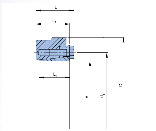
RINGFEDER® Anillos de contracción RfN 4161 • Dimensiones
